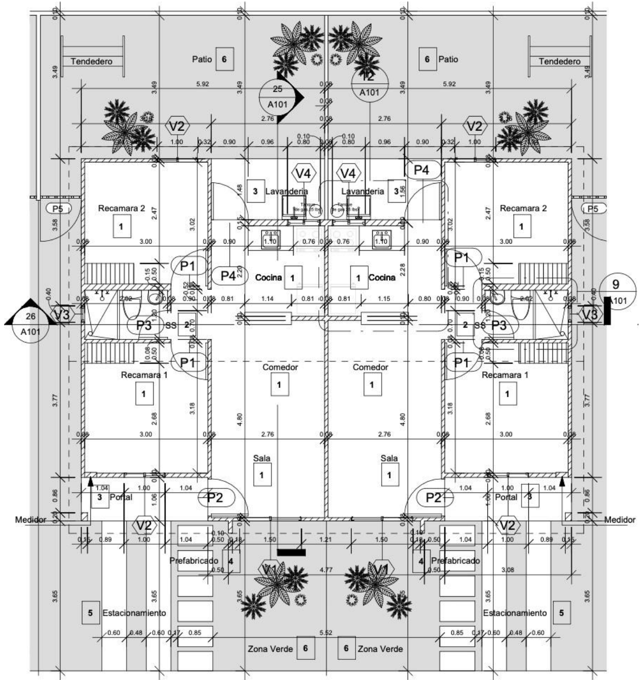
1 Planta Arquitectonica 1 : 75
